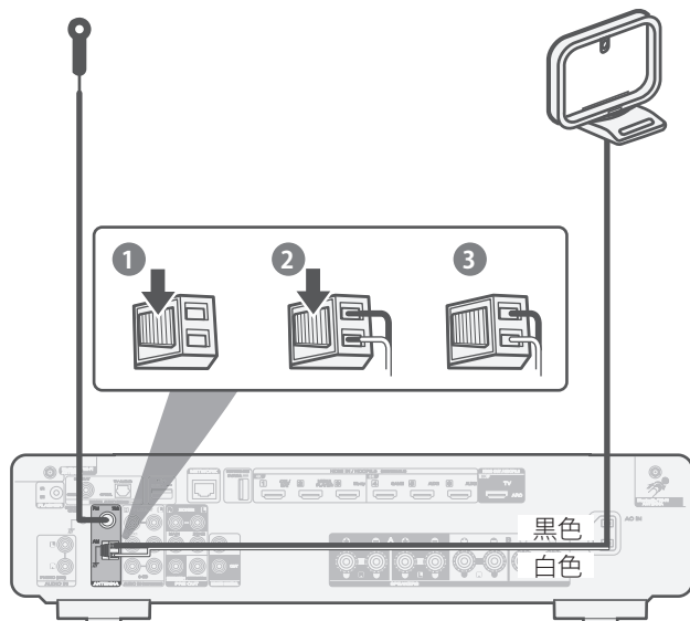
FM室内アンテナ (付属)
